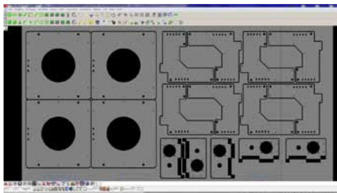
Nesting di punzonatura
